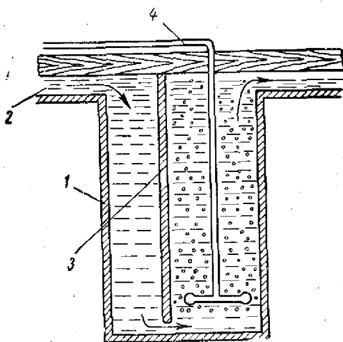
Рис. 79. Компрессорная воздухоподводящая система Г. Н. Парадня:
