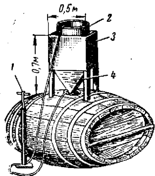
Рис. 120. Бочка овальной формы, оборудованная аэратором конструкции Трутня:
