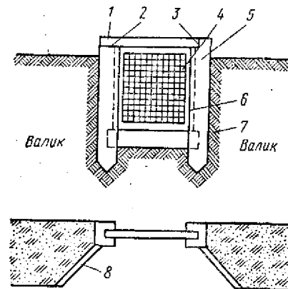
Рис. 93. Установка решетки в чеке:
