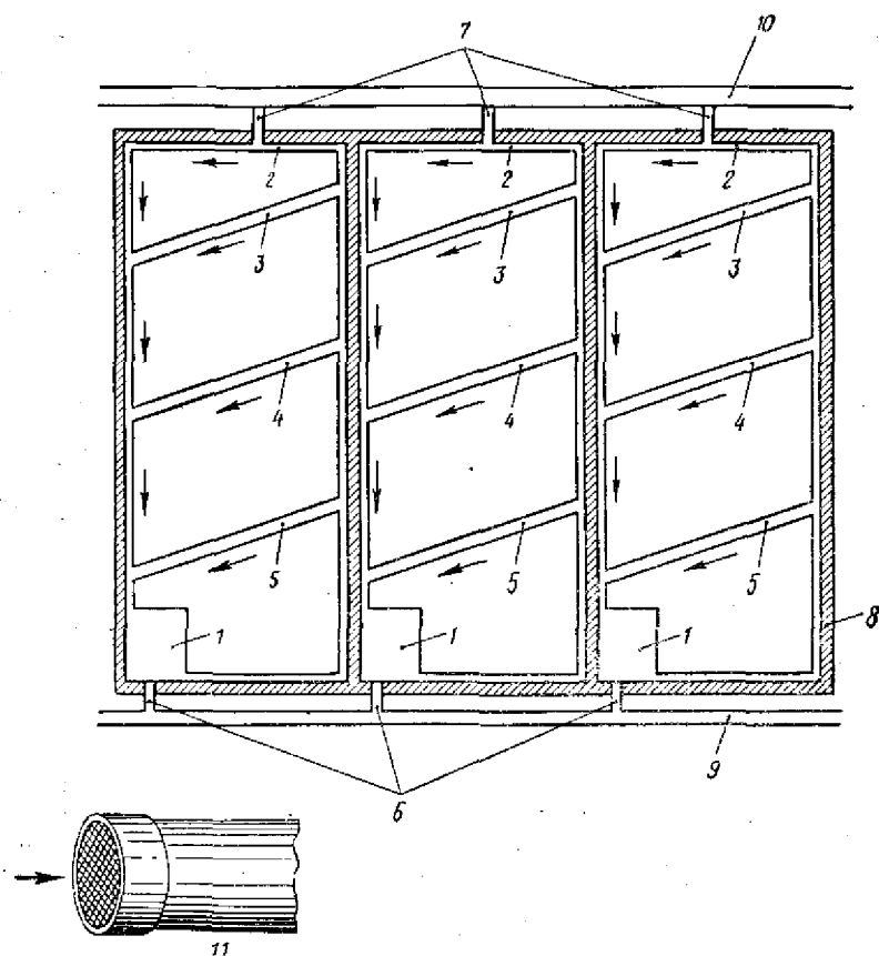
Рис. 92. План дна рисо-рыбных чеков:
