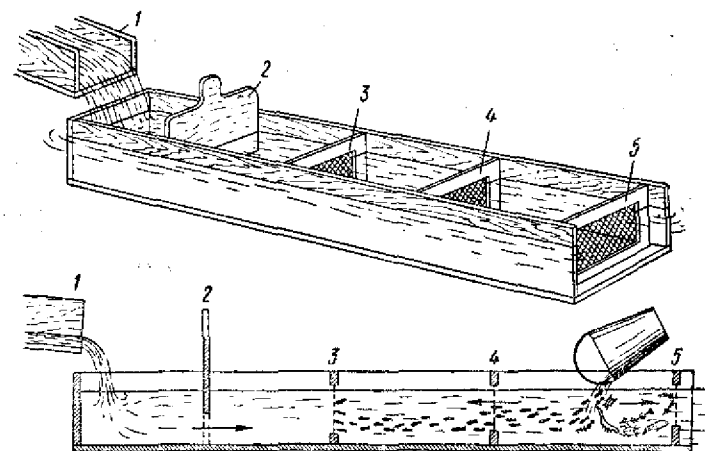
Рис. 30. Мальковый очиститель конструкции Т. Т. Соловьева:
