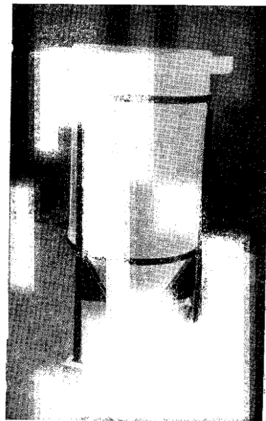
Рис. 73. Усовершенствованный аппарат ВНИИПРХа со стойкой для инкубации икры растительноядных рыб емкостью 100 л
