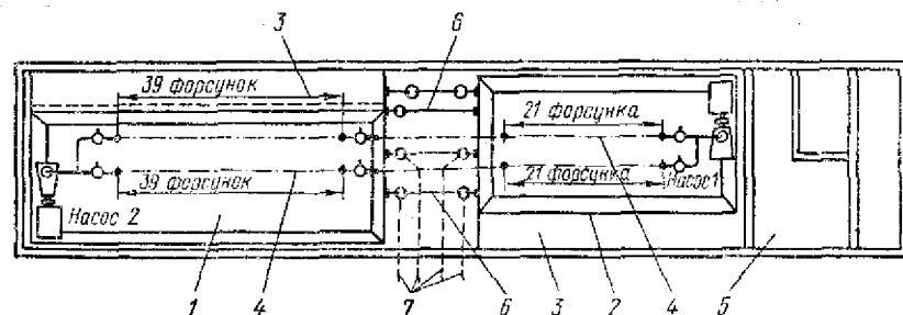
Рис. 122. Вагон с аэрационной установкой:
