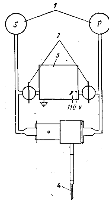
Рис. 105. Схема устройства для взятия икры при помощи воздуха:
