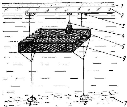
Рис. 113. Установка зимовального погружаемого садка для рыб, не нуждающихся в зимнем кормлении (на глубине 1—1,2 м):
