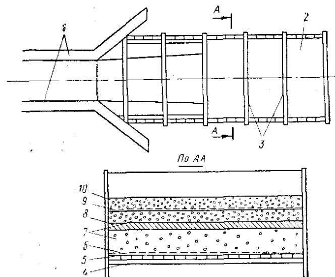
Рис. 84. Фильтр-уловитель сорной рыбы:
