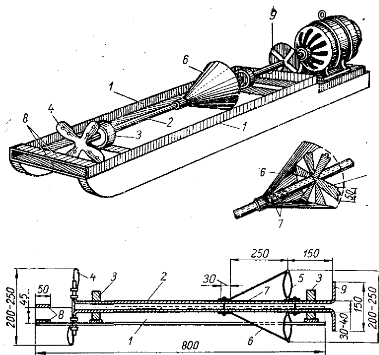
Рис. 77. Винтовой аэратор системы Т. Т. Соловьева:
