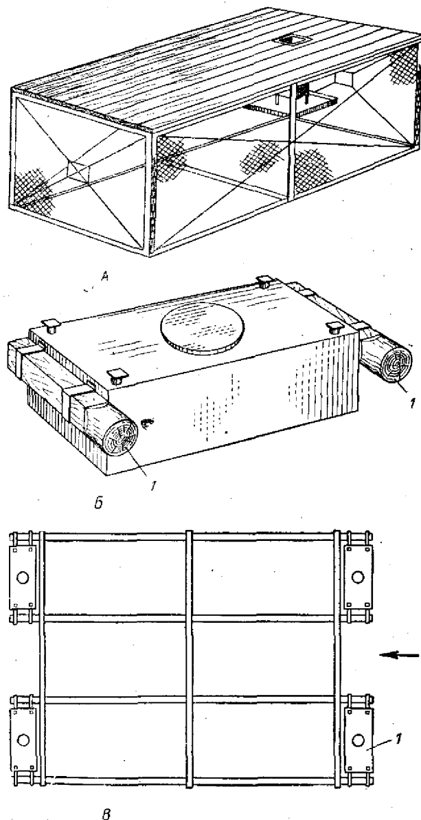
Рис. 90. А — вид садка с крышкой и кормовым столиком; Б — понтон садка и способ его крепления (1 — понтон); В — секция из 6 садков с четырьмя понтонками
