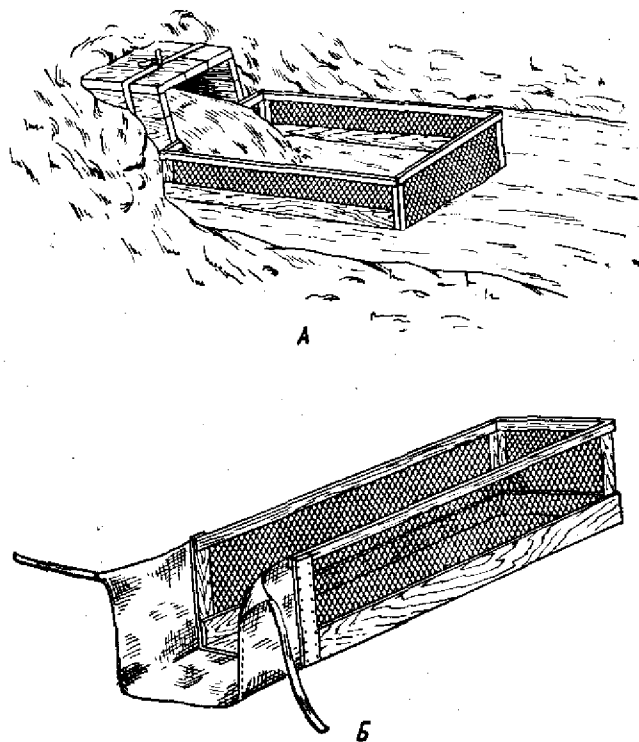
Рис. 29. Уловитель мальков. А — ящик-уловитель под концом лежака монаха в водосборной канаве; Б — брезентовый обплаг на конце уловителя для соединения с концом монаха
