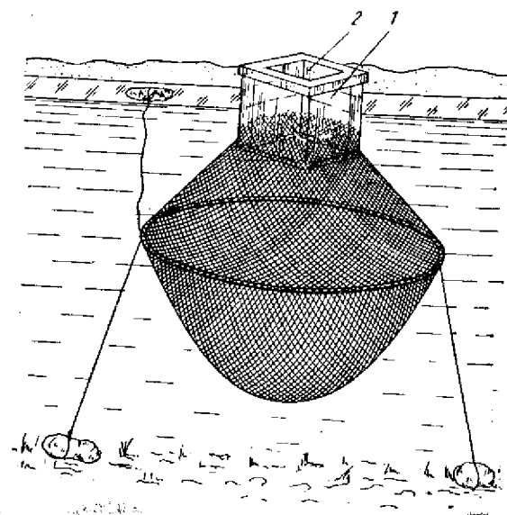
Рис. 112. Полупогружаемый садок для рыб, нуждающихся в зимнем кормлении (форель, сиг и др.):
