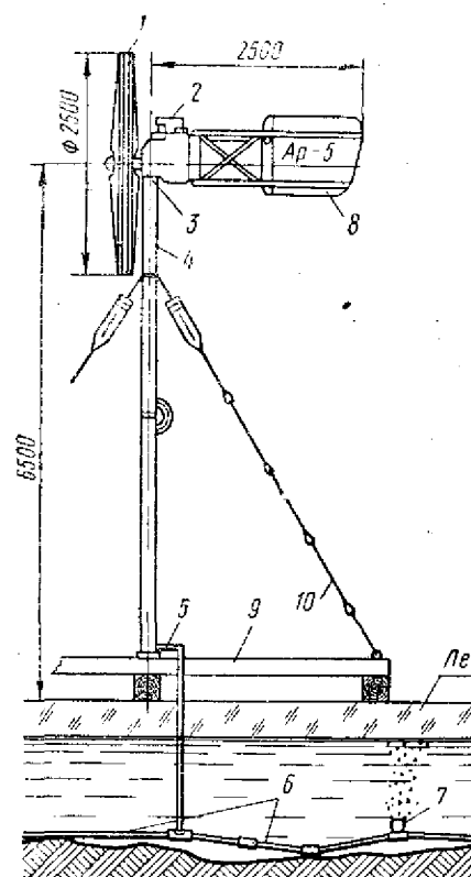
Рис. 78. Пневматический ветро-силовой аэратор для заморных водоемов (системы Решетникова).
