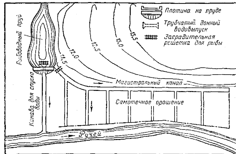
Рис. 99. Пруд атмосферного питания, предназначенный для рыборазведения и самотечного орошения
