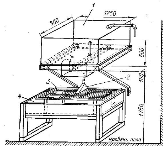
Рис. 107. Установка для отмывки икры: 1 — бак для воды, 2 — воронка душевая, 3 — транспортная рама, 4 — стол
