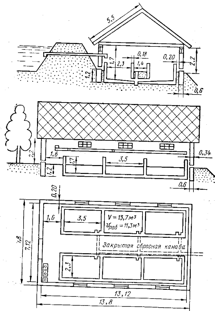
Рис. 37. Схема зимовального живорыбного домика с цементными бассейнами
