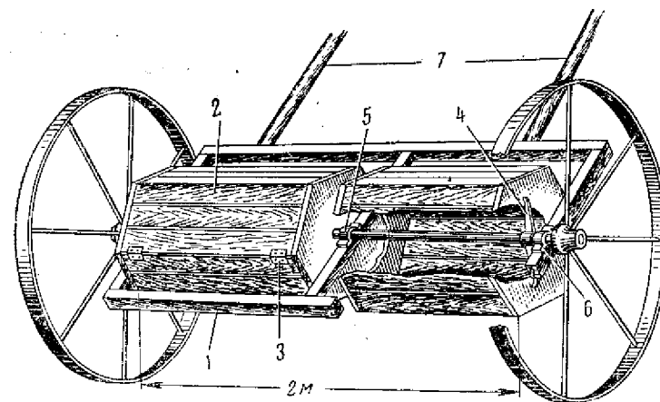
Рис. 83. Известковый барабан:
