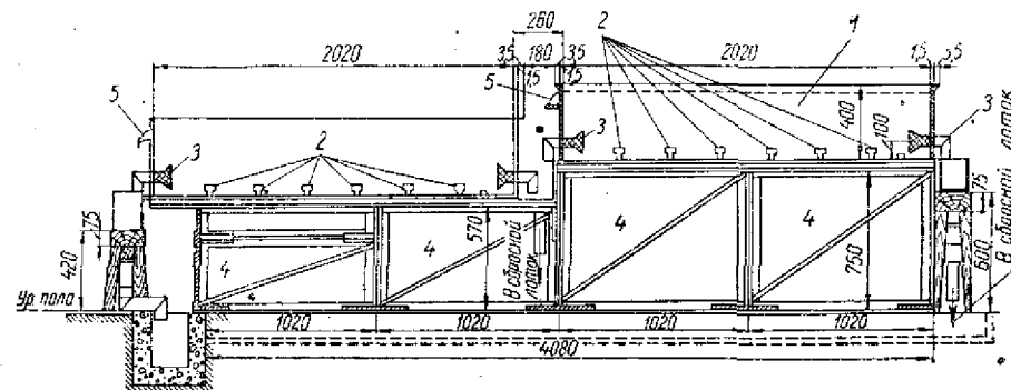
Рис. 109. Лоток системы Черфаса—Козлова для подращивания молоди форели: 1 — оцинкованный бассейн, 2 — сетчатые колпачки, 3 — водоспуски, 4 — стойка для установки оцинкованного бассейна, 5 — сливное окно
