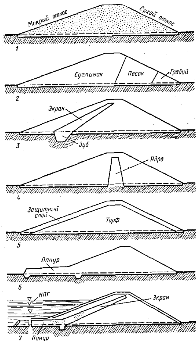
Рис. 19. Плотины из суглинистых и супесчаных грунтов: 1 — из однородного минерального грунта, 2 — из неоднородного минерального грунта, 3 — с экраном, 4 — с ядром, 5 — с применением торфа; 6 — с понуром, 7 — с экраном и понуром
